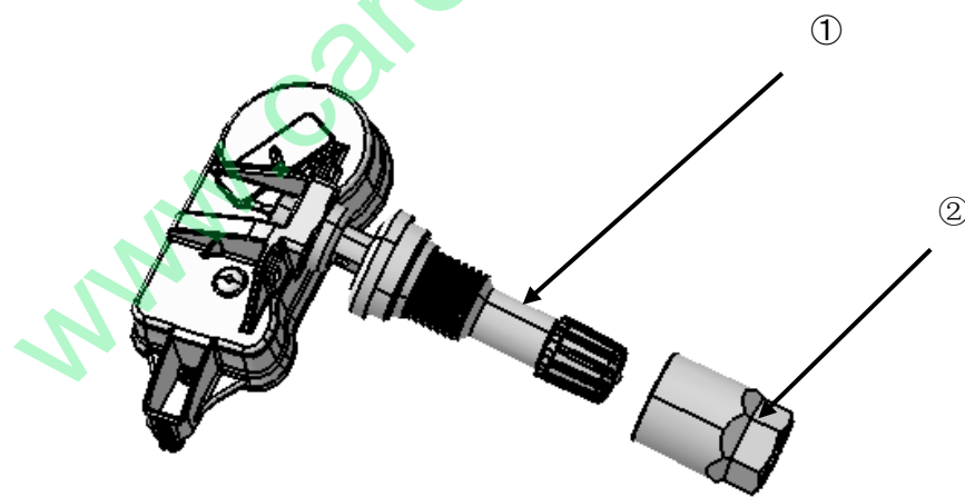
图 1.4 传感器拆分图
